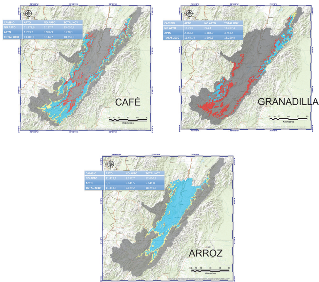
Figura 16. Proyecciones de cambio de aptitud de suelos para los cultivos café (A), granadilla (B) y arroz (C) debido al cambio climático para el período actual a 2030.
