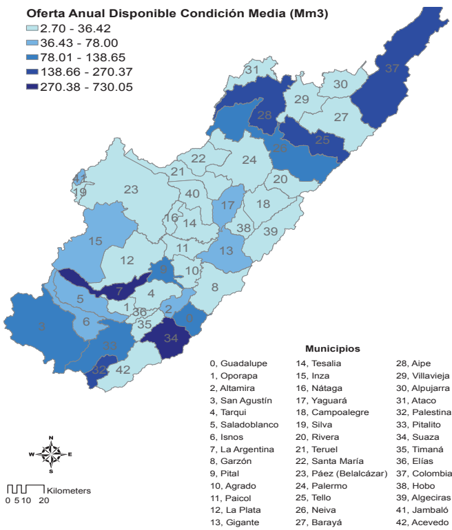
Figura 6. Oferta hídrica para la cuenca del Alto Magdalena, en condiciones climáticas medias (arriba) y secas (abajo) [en millones de metros 3 /año].
