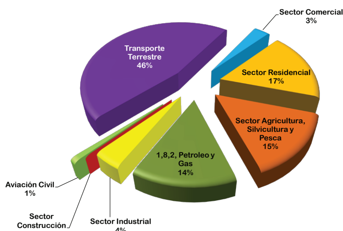
Figura 30. Emisiones por subsector: sector energía.
