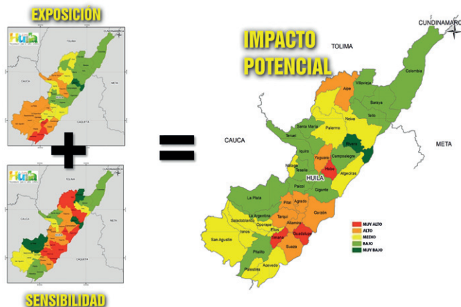
Figura 21. Impacto potencial del cambio climático en los municipios del Huila.
