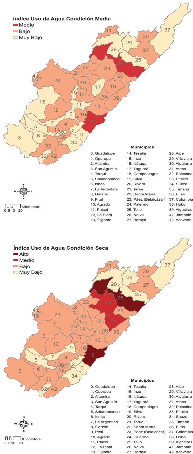
Figura 7. Índice de uso del agua para la condición climática media (arriba) y condición climática seca (abajo).
