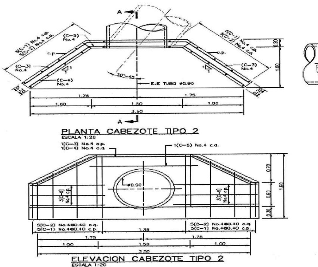
Figura 6 Planta cabezotes alcantarilla 36"
