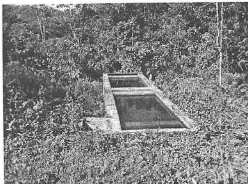
Fotografía 5. Desarenador.
