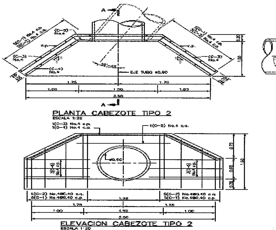
Figura 6 Planta cabezotes alcantarilla 36"
