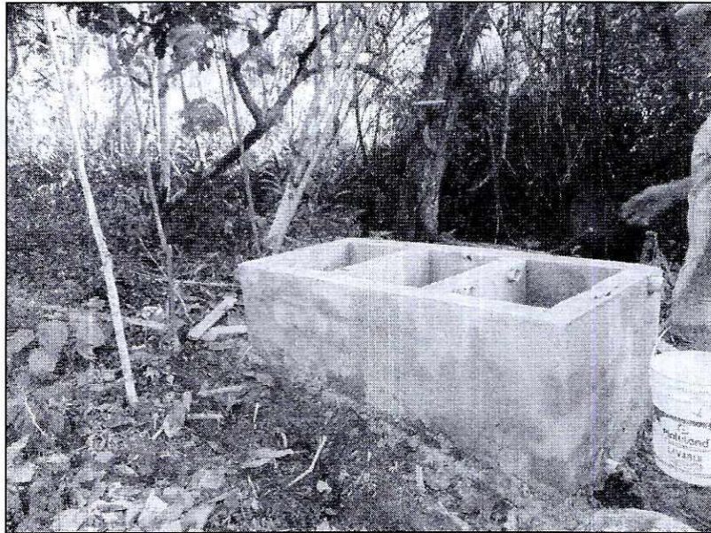
Desarenador del sistema de acueducto predio La Aurora.
