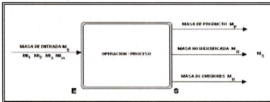
Figura 1. Esquema de entradas y salidas de un sistema para la evaluación por balance de masas.
